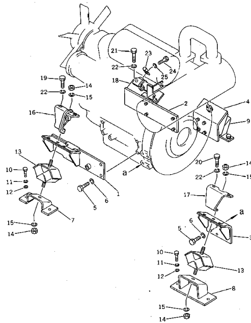
エンジン 取 付 部 品 Fig. 101 ENGINE MOUNTING PARTS
