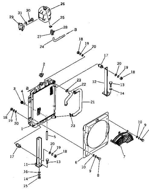
ラジエータ およびパイピング Fig. 131 RADIATOR AND PIPING
