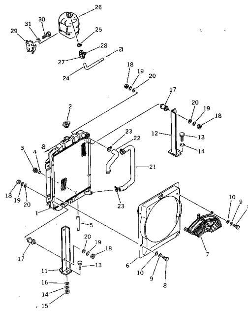
ラジエータ(適用機種) Fig. 131A RADIATOR (Serial No. 1668~)
