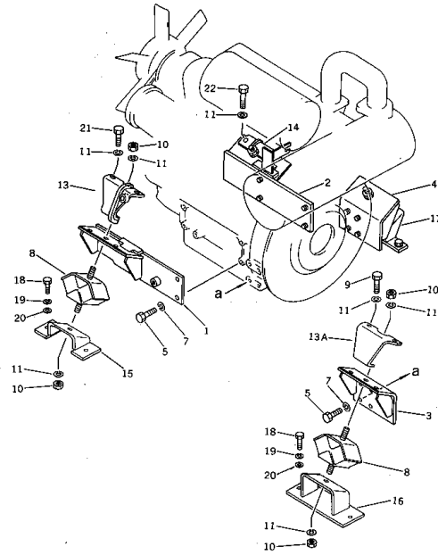
エンジン 取付 部品 Fig. 1101 ENGINE MOUNTING PARTS
