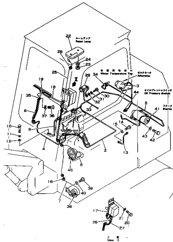
エレクトリカル システム Fig. 161 ELECTRICAL SYSTEM
