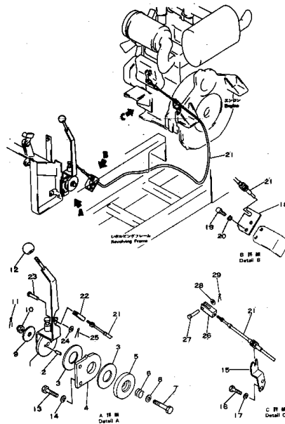
フュエルコントロール レバー Fig. 121 FUEL CONTROL LEVER
