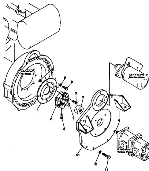
パワーテークオフ Fig. 105 POWER TAKE OFF
