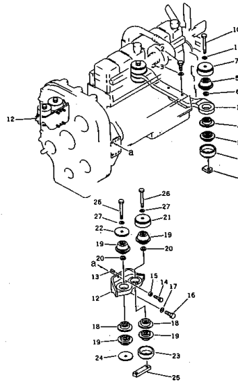
エンジン 取付 部品 品 S6D170 エンジン用 Fig. 1001A ENGINE MOUNTING PARTS (For S6D170 Engine) (適用 番 号 10007 ~ ) (Serial No. 10007 ~ )
