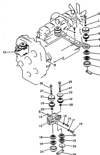
エンジン 取付部 図 KT1150 エンジン用 Fig. 1001 ENGINE MOUNTING PARTS (For KT1150 Engine) (適用 機種 Serial No. 10001 ~ 10006)
