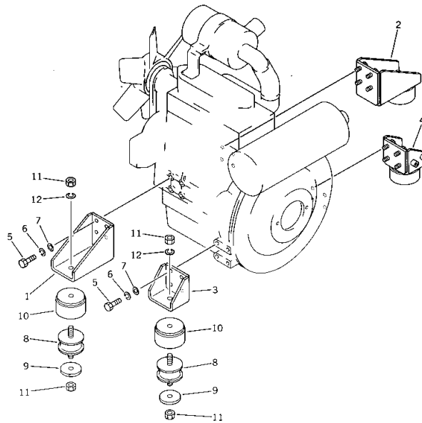
エンジン 取付 部品 FIG. 1001 ENGINE MOUNTING PARTS 適用機種 国内 向 (SERIAL NO. 2501-3100) (FOR JAPAN) 適用機種 海外 向 (SERIAL NO. 10401-10600) (EXCEPT JAPAN)
