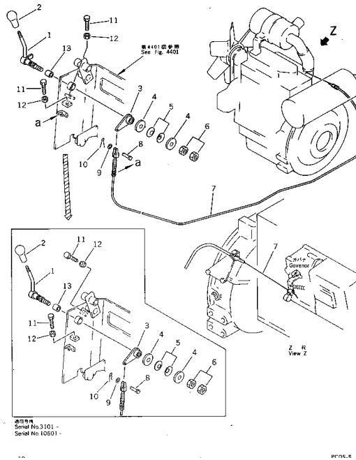
FIG. 1101 FUEL CONTROL LEVER 燃料コントロールレバー
