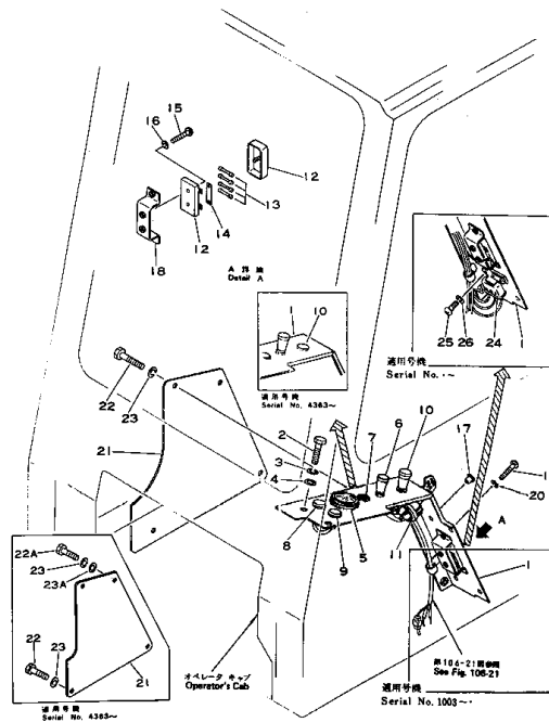
Fig. 105 インストルメント パネル および エレクトリカル システム INSTRUMENT PANEL AND ELECTRICAL SYSTEM
