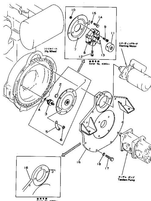
Fig. 102 パワー タイク オフ POWER TAKE OFF
