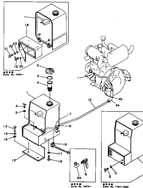
Fig. 104 FUEL TANK AND PIPING フエール タンク および パイピング
