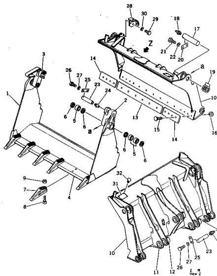
バケット Fig. 101 BUCKET
