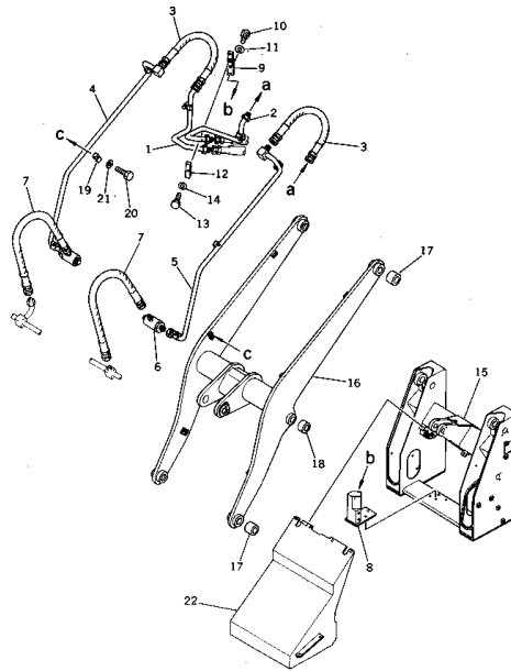
ハイドロリックパイピング Fig. 122 HYDRAULIC PIPING (2/3)
