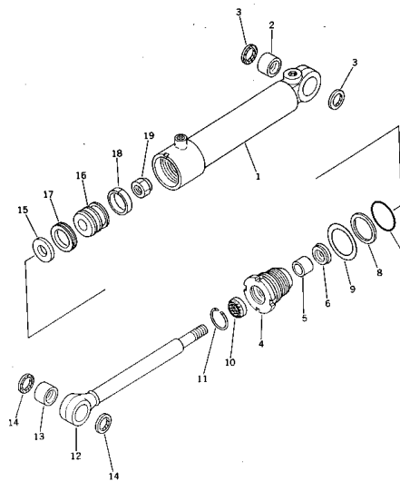
シリンダ Fig. 111 CYLINDER
