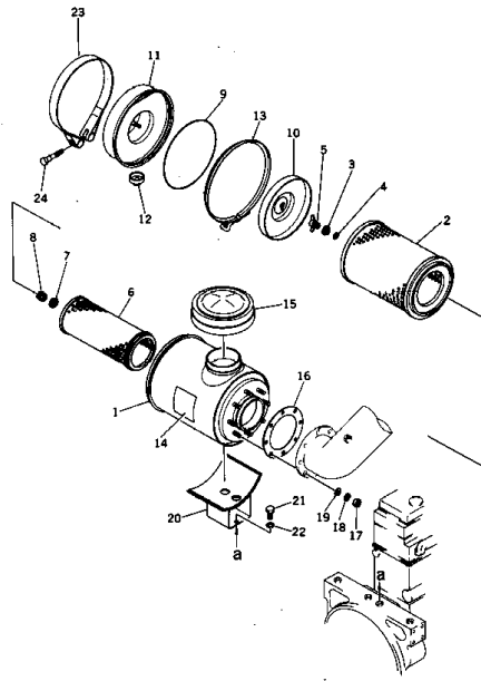
エアークリーナ および コネクション FIG. 117A AIR CLEANER AND CONNECTION
