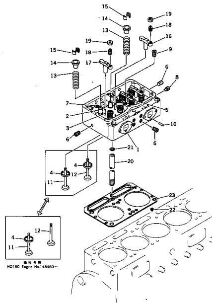
FIG. 101 シリンダヘッド CYLINDER HEAD
