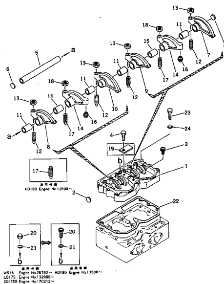
FIG. 103 ロッカーアームおよびハウジング ROCKER ARM AND HOUSING
