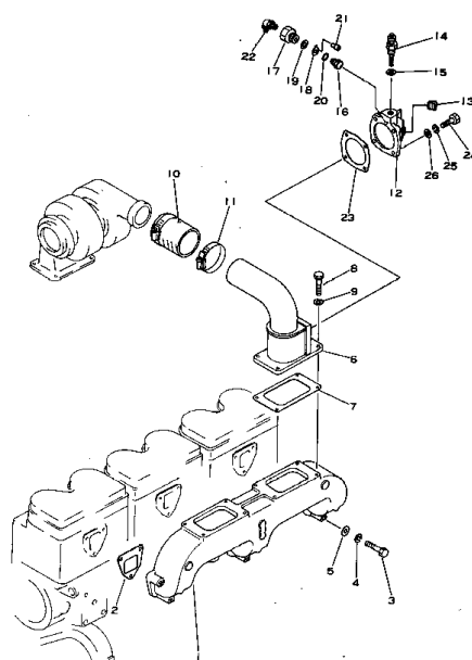
エア- インテーク マニホールド および コネクション FIG. 113 AIR INTAKE MANIFOLD AND CONNECTION
