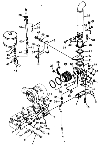
エキゾースト マニホールド および コネクション Fig. 121 EXHAUST MANIFOLD AND CONNECTION (WP22 Engine No. 108380~)
