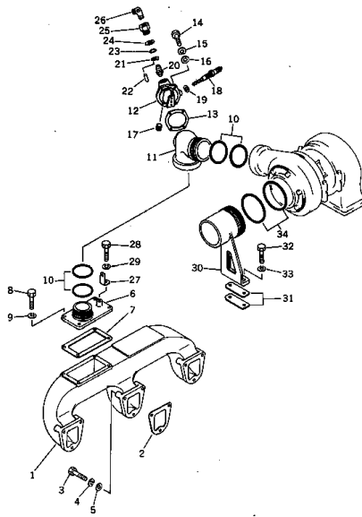
エア インテーク マニホールド および コネクション Fig. 111 AIR INTAKE MANIFOLD AND CONNECTION (適用 号 数 WF22 Engine No. 108380~)
