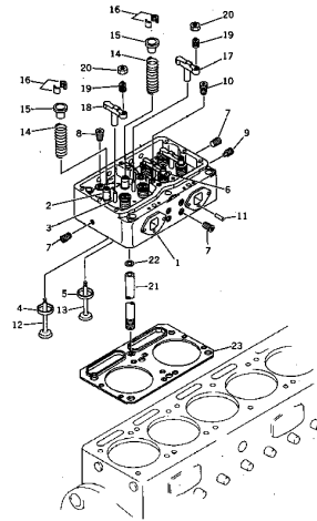
Fig. 101 シリンダ ヘッド CYLINDER HEAD
