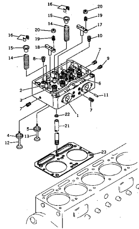
Fig. 101 シリンダヘッド CYLINDER HEAD
