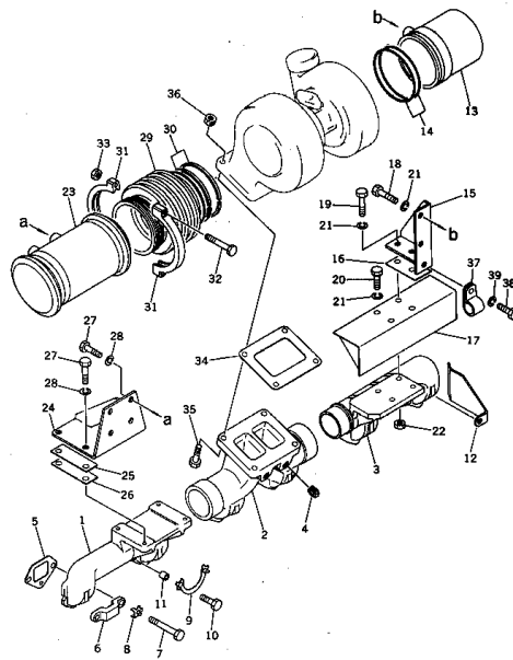
エキゾースト マニホールド および コネクション Fig.122 EXHAUST MANIFOLD AND CONNECTION (HD200 Engine No. 125628~147773)
