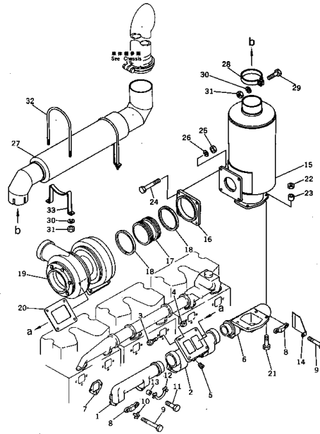
エキゾースト マニホールド および コネクション Fig. 124 EXHAUST MANIFOLD AND CONNECTION 適用 号 機 (EC260V Engine No. 134528~)
