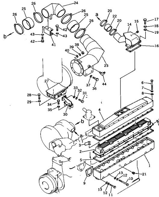
エアインテーク マニホールド および アフタ クーラ FIG. 0131 AIR INTAKE MANIFOLD AND AFTER COOLER
