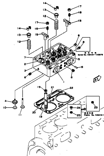
シリンダヘッド FIG. 1101 CYLINDER HEAD
