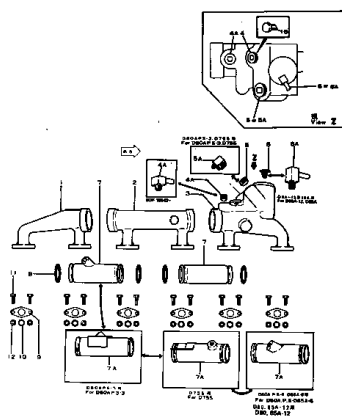
ウォーター マニホールド Fig. 109 WATER MANIFOLD
