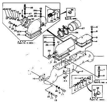
Fig. 114 エアー インテーク マニホールド および コネクション AIR INTAKE MANIFOLD AND CONNECTION (GD37 Engine No. 1926~)
