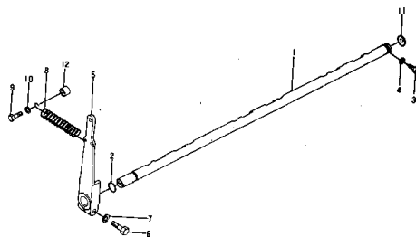
Fig. 108 コンプレッション リリース (適用機種 GD37 Engine No. 1926~)
