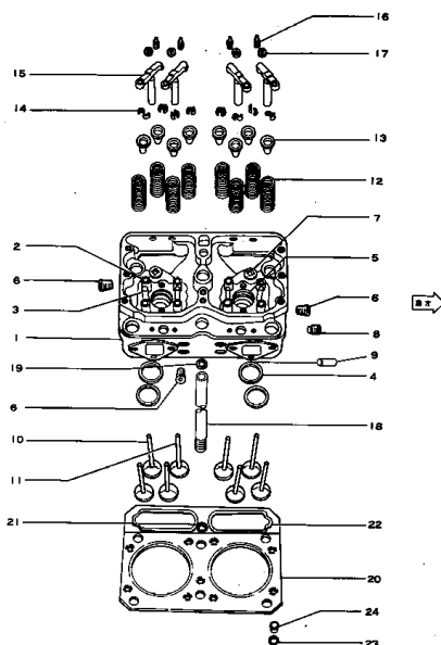
Fig. 101 シリンダヘッド CYLINDER HEAD
