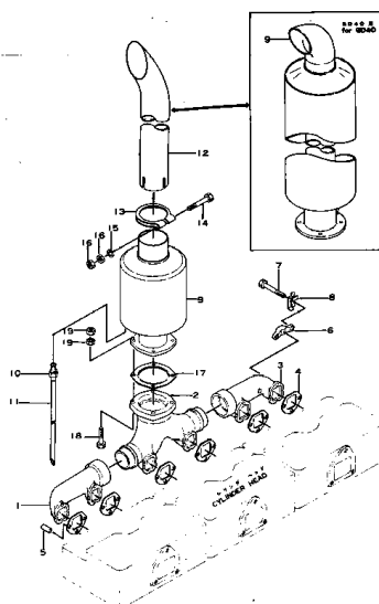
エキゾースト マニホールド および マフラー Fig. 119 EXHAUST MANIFOLD AND MUFFLER (GD37,GD40 適用 機種 Engine No. 1926~)
