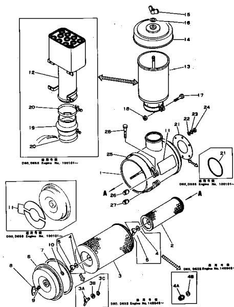
エアー クリーナ 構造図 FIG. 1115 AIR CLEANER (ENGINE NO. 100101 ~ 139166)
