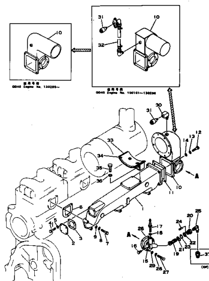
エアインテークマニホールドおよびコネクション FIG. 1114 AIR INTAKE MANIFOLD AND CONNECTION
