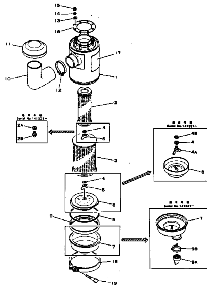
エアークリーナ FIG. 1117 AIR CLEANER
