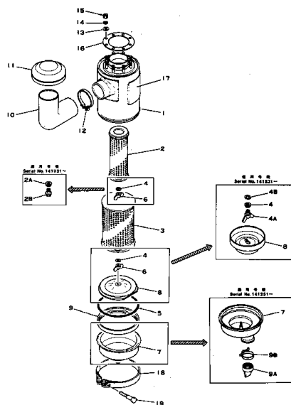
エアークリーナー FIG. 1117 AIR CLEANER
