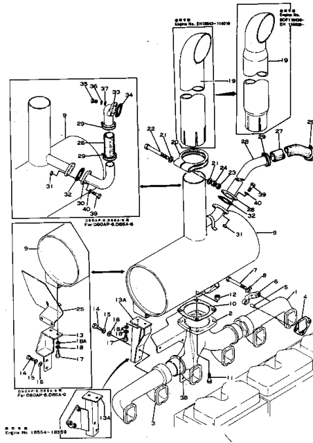
エキゾースト マニホールド および マフラー FIG. 115B EXHAUST MANIFOLD AND MUFFLER
