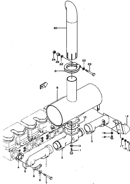
エキゾースト マニホールド および マフラ 適用号 FIG. 117 EXHAUST MANIFOLD AND MUFFLER (ENGINE NO. 8289—11295)
