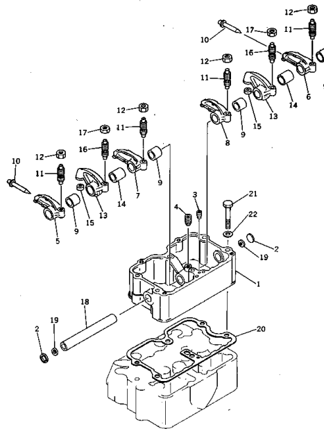
Fig. 103 ロッカーアームおよびハウジング ROCKER ARM AND HOUSING
