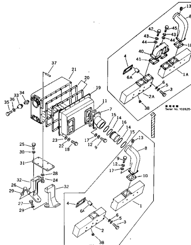
Fig. 111 エア インテーク マニホールド および コネクション AIR INTAKE MANIFOLD AND CONNECTION
