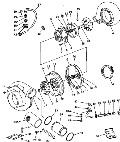
ターボチャージャー (機用号機) Fig. 141 TURBOCHARGER (Engine No. 103559-103924)
