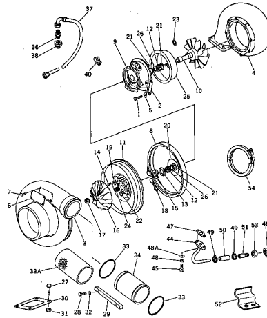
ターボチャージャー (エンジン No. 103925~) Fig. 141A TURBOCHARGER (Engine No. 103925~)
