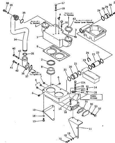
FIG. 135 THERMOSTAT (ENGINE NO. 117097-122721)
