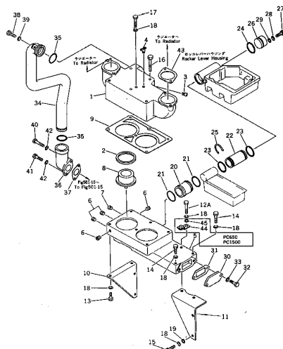
サーモスタット 適用図 FIG. 135 THERMOSTAT (ENGINE NO. 101153-122721)
