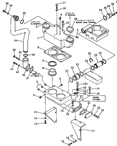
サーモスタット 適用 図 FIG. 135 THERMOSTAT (ENGINE NO. 117097 - 122721)
