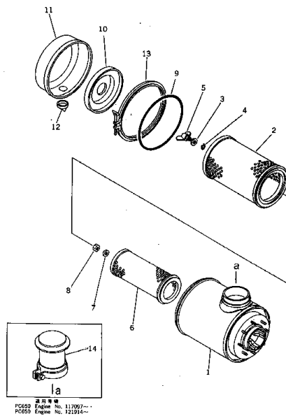
エアークリーナ FIG. 116 AIR CLEANER
