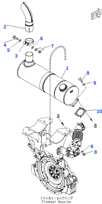
フライホイールハウジング Flywheel Housing
