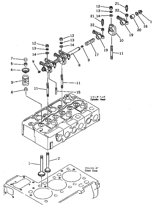
ロッカ アーム、インレット および エキゾースト バルブ Fig. 107 ROCKER ARM, INLET AND EXHAUST VALVES
