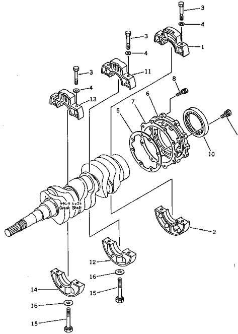
メイン ベアリング ケース Fig. 105 MAIN BEARING CASE
