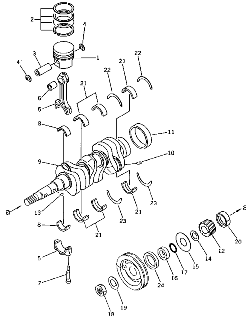
ピストンおよびクランクシャフト Fig. 111 PISTON AND CRANKSHAFT
