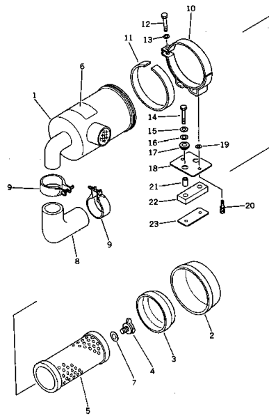
エアークリーナ Fig. 105 AIR CLEANER
