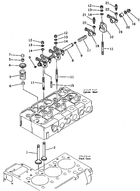
Fig. 102 ロッカーアーム、インレットおよび エキゾーストバルブ ROCKER ARM, INLET AND EXHAUST VALVES
