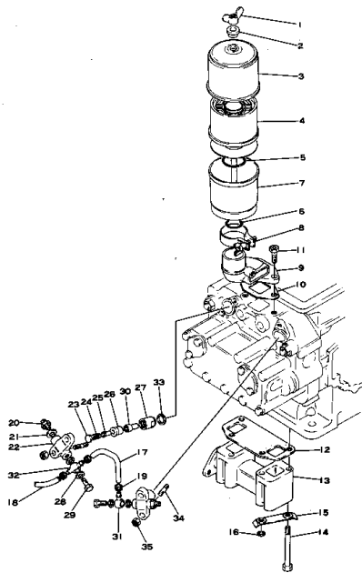
Fig. 107 エアークリーナおよびエキゾースト マニホールド AIR CLEANER AND EXHAUST MANIFOLD
