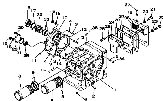
Fig. 101 クランクケース CRANKCASE
