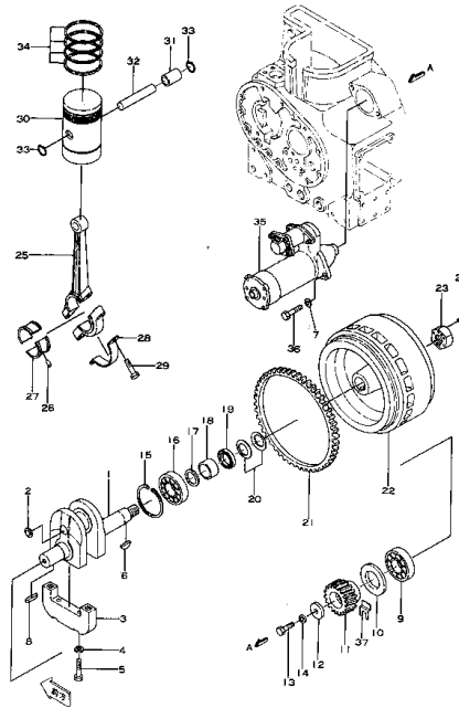
クランクシャフト、ピストン、フライホイール および スタータ Fig. 106 CRANKSHAFT, PISTON, FLYWHEEL AND STARTER
