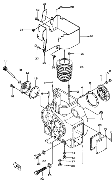
シリンダ ブロック Fig. 104 CYLINDER BLOCK
