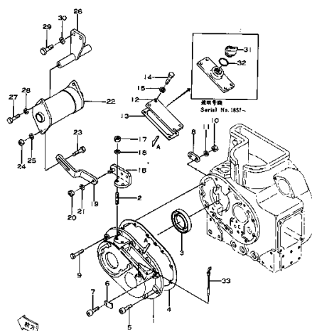
ギヤケース (適用機種) Fig. 105 GEAR CASE (Serial No. 1385~)
