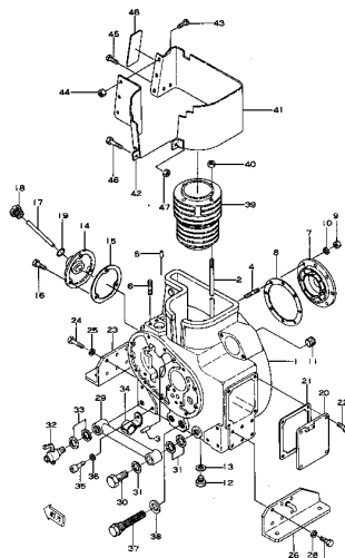
Fig. 104 CYLINDER BLOCK (適用機種 (Serial No. 1385-))
