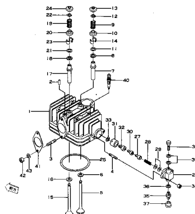
Fig. 101 シリンダヘッドおよびノズルホルダ CYLINDER HEAD AND NOZZLE HOLDER (適用機種 Serial No. 1385~)
