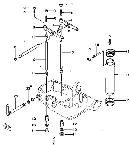
ロ ッ カ アーム および プッシュ ロッド (適用 号 機) Fig. 102 ROCKER ARM AND PUSH ROD (Serial No. 1385~)
