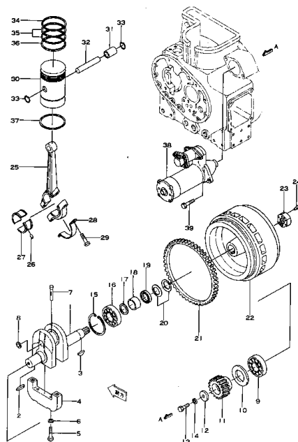
Fig. 106 クランクシャフト、ピストン および フライホイール CRANKSHAFT, PISTON AND FLYWHEEL (適用 号 機 Serial No. 1385~)
