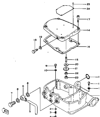
Fig. 103 ROCKER ARM HOUSING (適用 機種 Serial No. 1385~)
