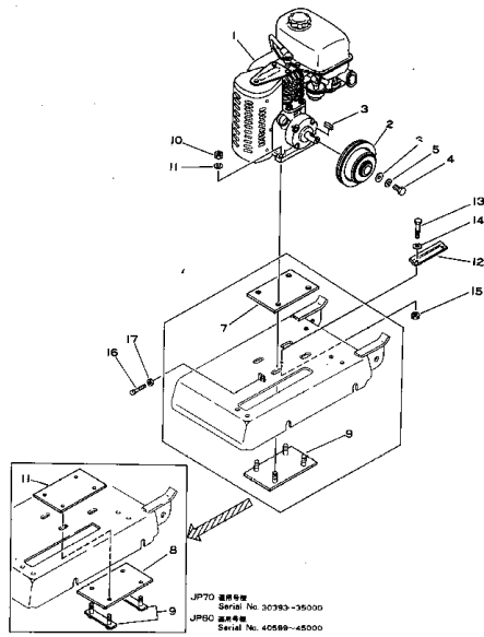
Fig. 101 ENGINE MOUNT (エンジンマウント) (適用機種) (JP70 Serial No. 30001~35000) (JP80 Serial No. 40001~45000)
