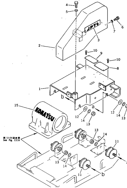
エンジンベースカバー (適用機種 Fig. 121B ENGINE BASE COVER (JP70 Serial No. 37001~) (JP80 Serial No. 47001~))
