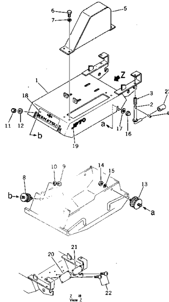
エンジンベースカバー (適用機種 Fig. 121A ENGINE BASE COVER (JP70 Serial No. 35001~37000) (JP80 Serial No. 45001~47000)
