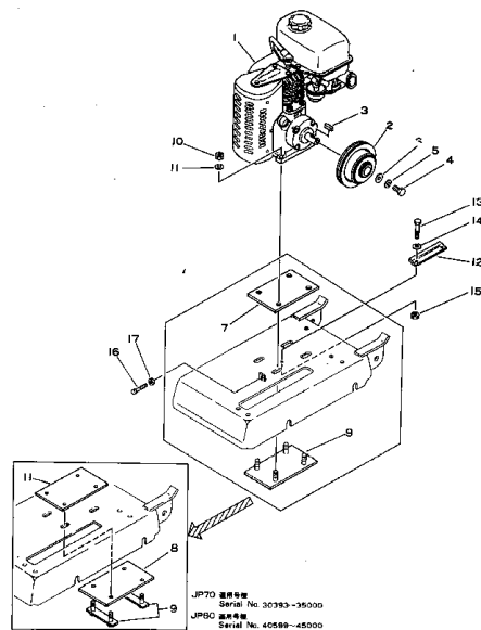
エンジンマウント (通称機種) Fig. 101 ENGINE MOUNT (JP70 Serial No. 30001~35000) (JP80 Serial No. 40001~45000)
