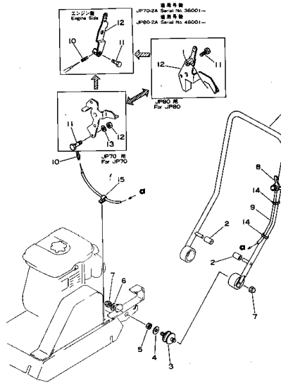
ハンドル (通用機種) Fig. 111A HANDLE (JP70 Serial No. 350001~37000) (JP80 Serial No. 450001~47000)
