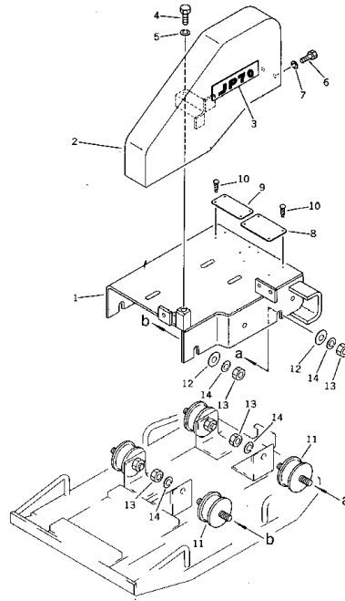
エンジンベースカバー (JP70 Serial No. 37001~) Fig. 121B ENGINE BASE COVER (JP80 Serial No. 47001~)
