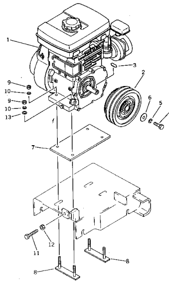
エンジンマウント (適用機種 JP70 Serial No. 37001~ JP80 Serial No. 47001~) Fig. 101B ENGINE MOUNT
