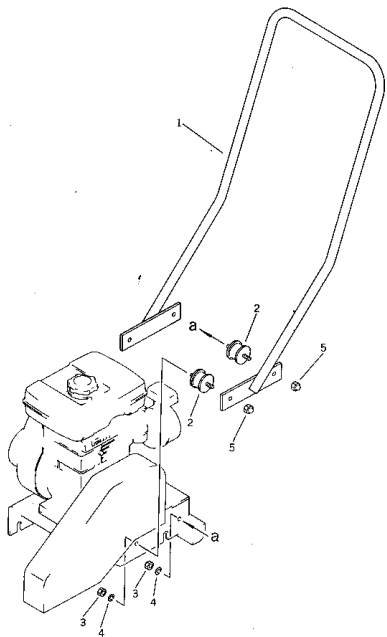
ハンドル (適用機種) Fig. 111B HANDLE (JP70 Serial No. 37001~) (JP80 Serial No. 47001~)
