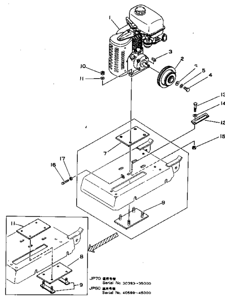
エンジンマウント (JP70 Serial No. 30001~35000) Fig. 101 ENGINE MOUNT (JP80 Serial No. 40001~45000)
