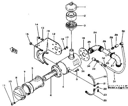
エアークリーナ (適用号機) Fig.113 AIR CLEANER (Serial No.0003~)
