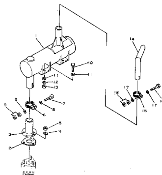
エキゾースト マフラー Fig. 111 EXHAUST MUFFLER
