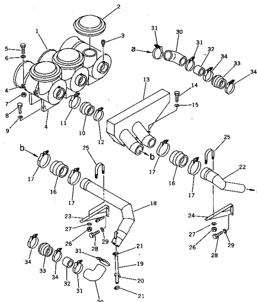
エア- インテーク パイピング カミンズ エンジン 用 FIG. 1033 AIR INTAKE PIPING (FOR CUMMINS ENGINE)
