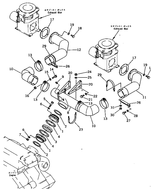
エキゾースト パイピング ボディーヒーティング機 FIG. 1041 EXHAUST PIPING (1/2) (WITH BODY HEATING) 小形エンジン用 (FOR KOMATSU ENGINE)
