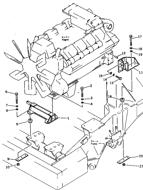
エンジン 取付部品 (FOR KOMATSU ENGINE) FIG. 1001 ENGINE MOUNTING PARTS (FOR KOMATSU ENGINE) 適用台数 (SERIAL NO. 1501-1528)
