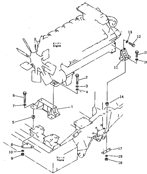
エンジン 取付 部品 カミンズエンジン用 FIG. 1005 ENGINE MOUNTING PARTS (FOR CUMMINS ENGINE)
