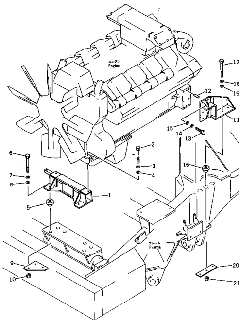
エンジン 取付部品 小松エンジン用 FIG. 1001A ENGINE MOUNTING PARTS (FOR KOMATSU ENGINE) 適用機種 (SERIAL NO. 1529-)
