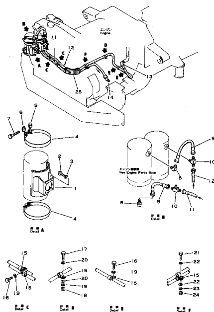
Fig. 107 バイパス フィルタ パイピング BYPASS FILTER PIPING
