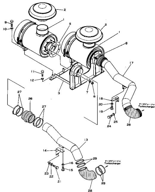
エア- インテーク システム (適用 号 機 1002~1026,1030,1034~1050) Fig. 116 AIR INTAKE SYSTEM (Serial No. 1037~1061,1066~1068)
