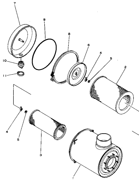
Fig. 115 エアークリーナ (適用機種 AIR CLEANER (Serial No. 1002~1033))
