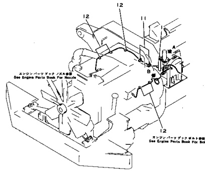
クイック スタート システム Fig. 114 QUICK START SYSTEM
