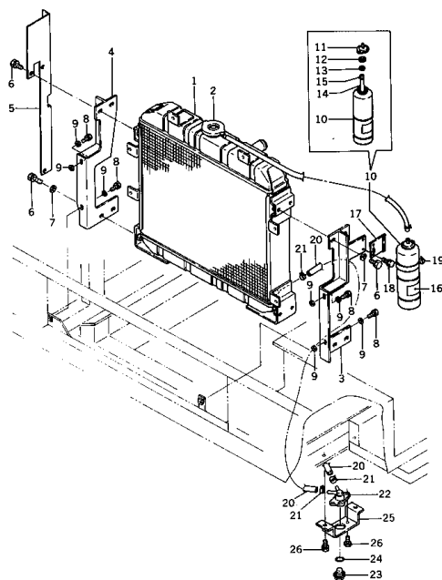
ラジエーター および 取付 部品 FIG. 1201 RADIATOR AND MOUNTING PARTS
