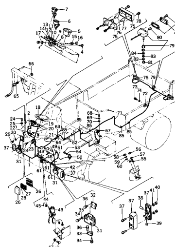
FIG. 1421 エレクトリカル システム ELECTRICAL SYSTEM
