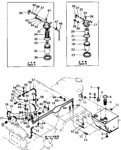
FIG. 1301 FUEL TANK AND PIPING フュエル タンク および パイピング
