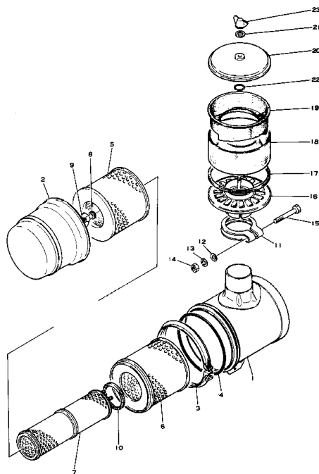
Fig. 1104 AIR CLEANER (Serial No. 0510~0725)
