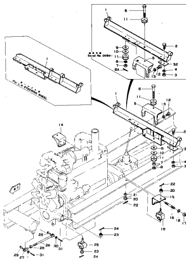
エンジン 取付 部品 Fig. 101 ENGINE MOUNTING PARTS
