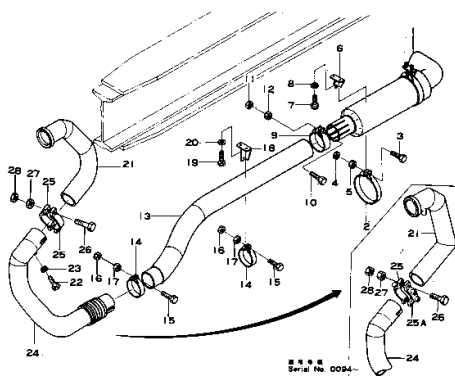
エキゾースト マフラー Fig. 102 EXHAUST MUFFLER
