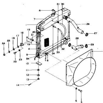
ラジエータ Fig. 104 RADIATOR
