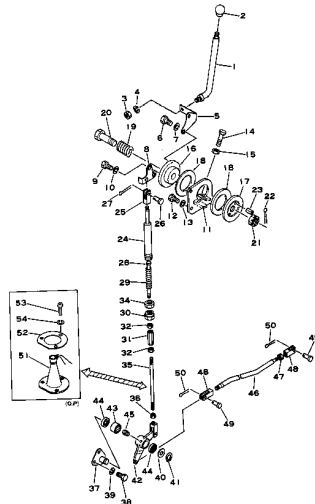
Fig. 1121 アー セ ル レバ ー Fig. 1121 ACCELERATOR LEVER
