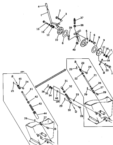
スロットル レバー リンケージ 適用機種 FIG. 122 THROTTLE LEVER LINKAGE (GD605A SERIAL NO. 54001 - )
