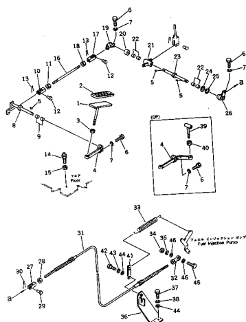
スロットル ペダル リンケージ 適用機種 FIG. 126A THROTTLE PEDAL LINKAGE (GD605A SERIAL NO. 54004 -)
