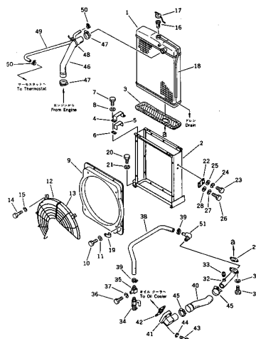
FIG. 131 RADIATOR
