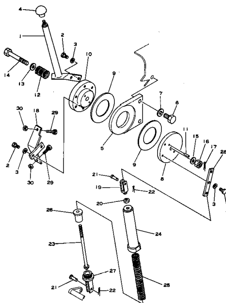
スロットル レバー リンケージ Fig. 121 THROTTLE LEVER LINKAGE
