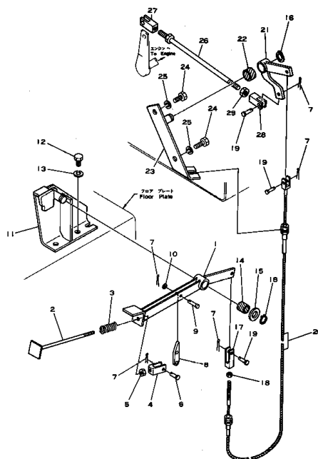
コンプレッション リリース レバー Fig. 111 COMPRESSION RELEASE LEVER
