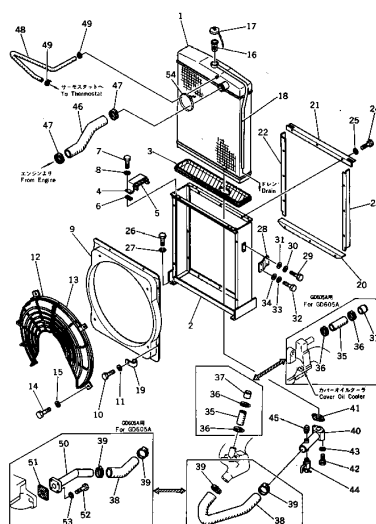
Fig. 131 RADIATOR
