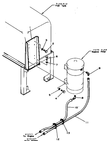
Fig. 102 バイパス フィルタ マウンティング Fig. 102 BYPASS FILTER MOUNTING
