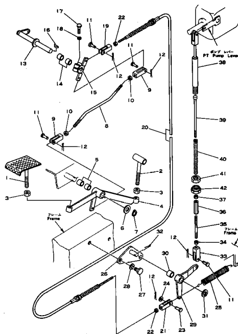
スロットル ペダル リンケージ Fig. 112 THROTTLE PEDAL LINKAGE
