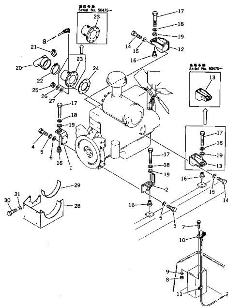
エンジン 取 付 部 品 Fig. 101 ENGINE MOUNTING PARTS
