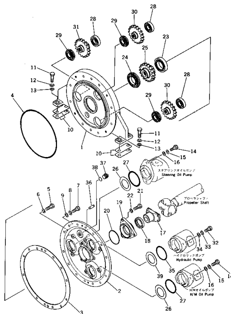
パワー テーク オフ Fig. 105 POWER TAKE OFF
