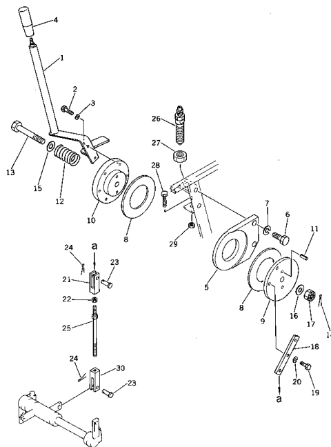
Fig. 122 FUEL CONTROL LEVER LINKAGE フエール コントロール レバー リンケージ
