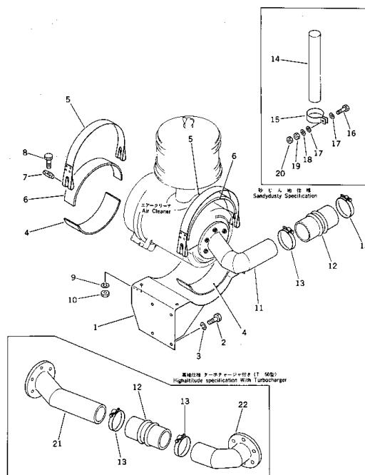
エアークリーナ ブラケット Fig. 113 AIR CLEANER BRACKET
