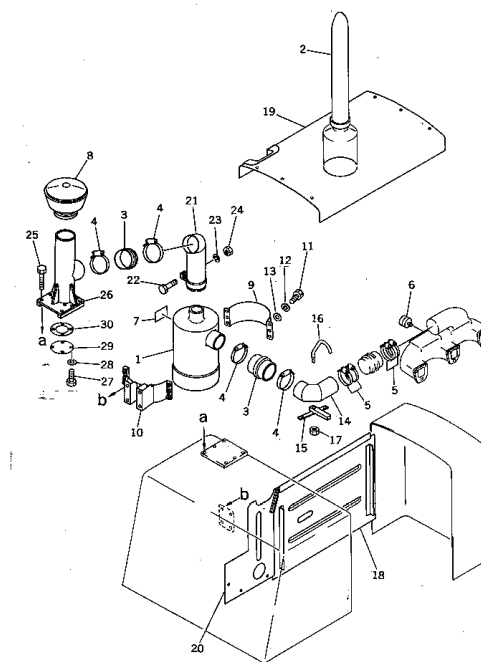
エアークリーナ オイルバス タイプ Fig. 114 AIR CLEANER OIL BAS TYPE (海外向) (適用番號 (Except Japan) (Serial No. 3705~)
