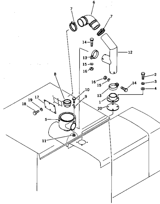
エアークレークダクト (適用機種) Fig. 117 AIR INTAKE DUCT(OP) (Serial No. 3705~)
