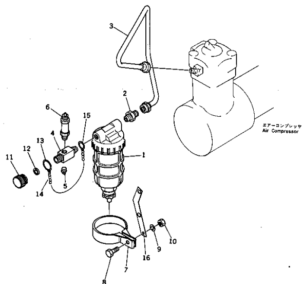
コンプレッサー エアークリーナ およびパイピング Fig. 104A COMPRESSOR AIR CLEANER AND PIPING(OP) (適用機種 Serial No. 4945~)
