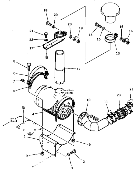
エアークリーナ カバー (通用機種) Fig. 115 AIR CLEANER COVER(OP) (Serial No. 4137~)
