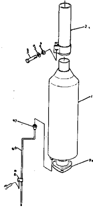
エキゾースト マ フ ラ (組 立 号 機) Fig. 111 EXHAUST MUFFLER (Serial No. 1003~1257)
