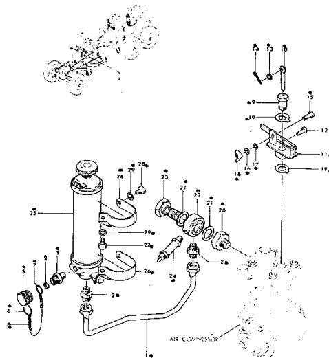
Fig. 113A コンプレッサ エアークリーナ およびパイピング COMPRESSOR AIR CLEANER AND PIPING (For Komatsu Engine Serial No. 1253~1327)
