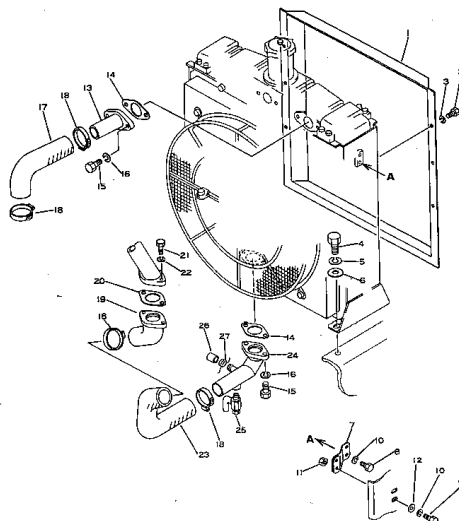
ラジエータ (高規格機) Fig. 111B RADIATOR(2/2) (Serial No. 4001~)
